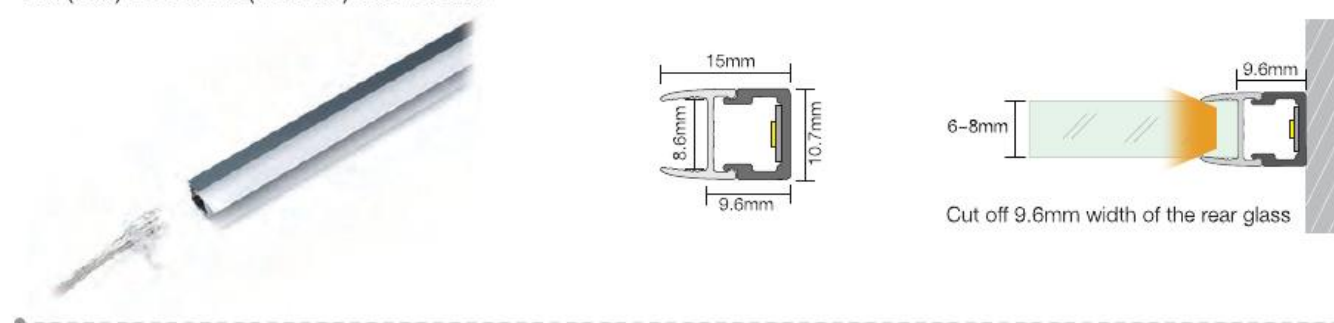
QC03A osvetlitev steklenih polic 12V (150 LED) & 24V(200LED)-10W-CRI 90+
