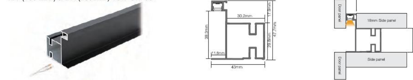
QC09B LED svetilka osvetlitev korpusa 12V (150 LED) & 24V(200LED)-10W-CRI 90+
