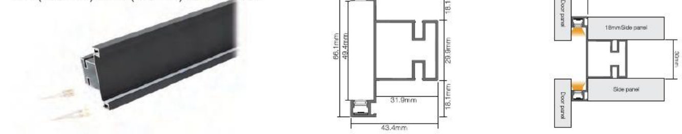
QC10B LED svetilka osvetlitev korpusa 12V (150 LED) & 24V(200LED)-10W-CRI 90+
