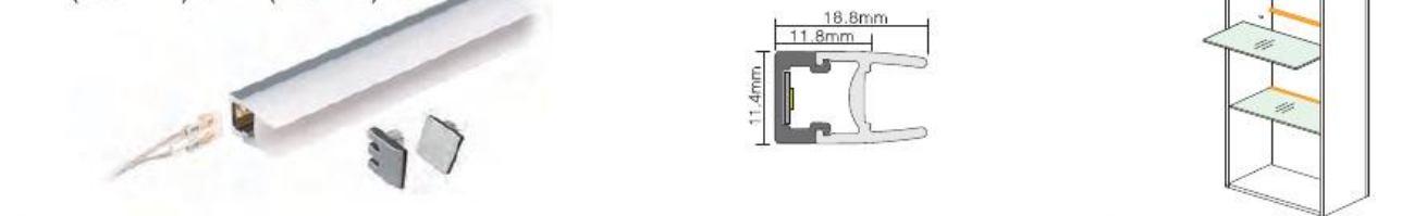
QC04B Svetilka za osvetlitev steklenih polic 12V (150 LED) & 24V(200LED)-10W-CRI 90+
